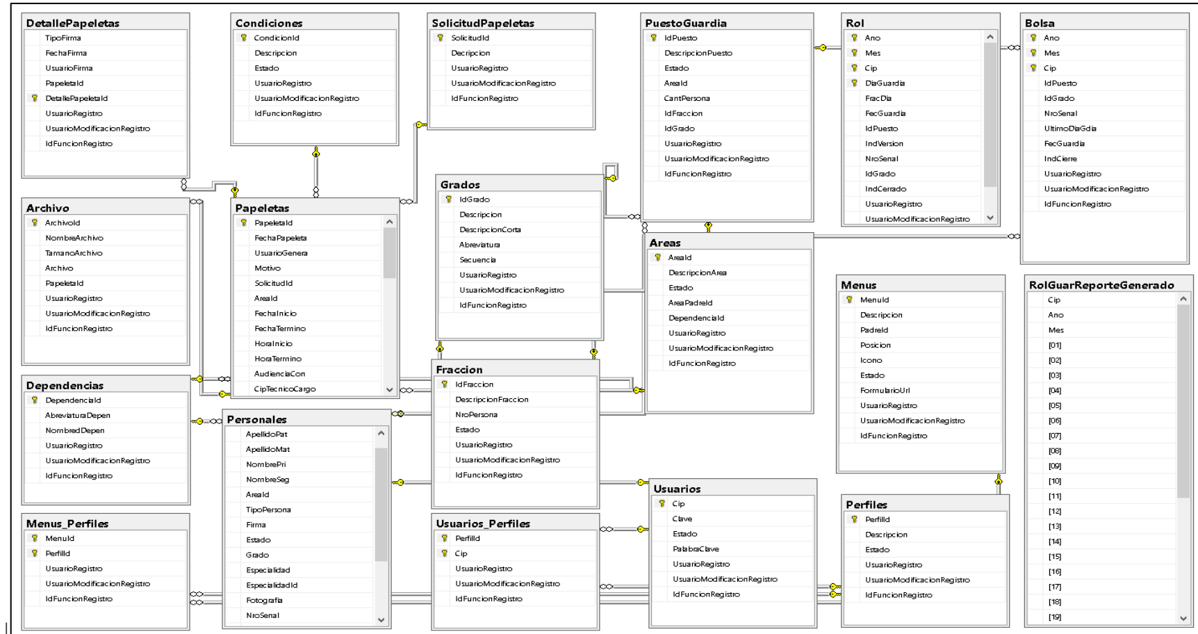
Ilustración 81 - Modelo de datos físico del sistema
