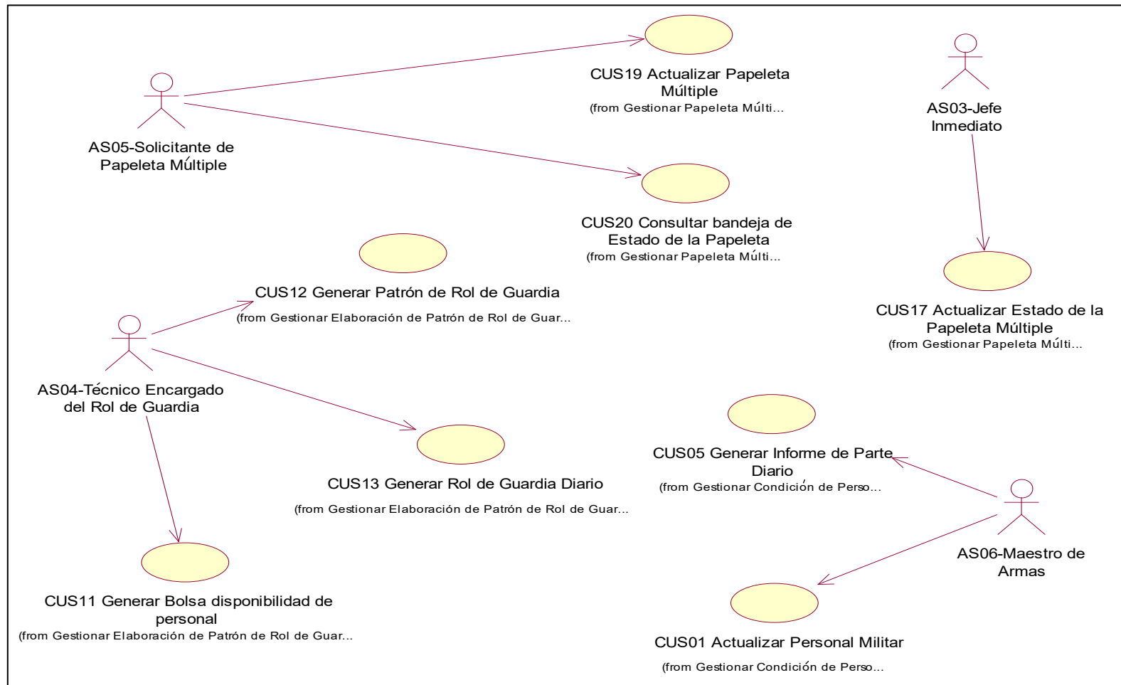
Ilustración 75 - Diagrama de casos de uso más significativos
