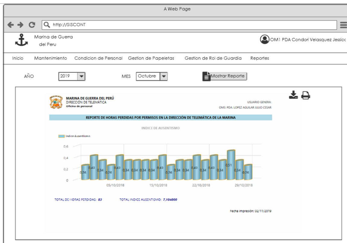
Ilustración 27 - Interfaz Reporte de índice de ausentismo Fuente: Elaboración Propia
