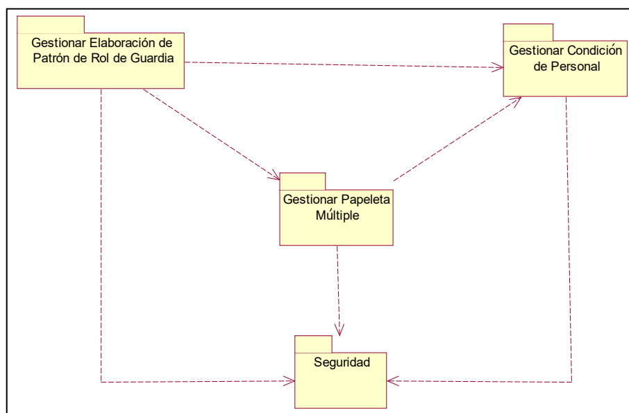
Ilustración 20- Diagrama de paquetes del sistema Fuente: Elaboración propia
