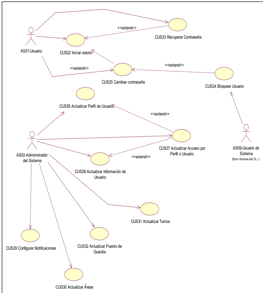
Ilustración 24-Diagrama de casos de uso del Sistema de Seguridad Fuente: Elaboración propia.
