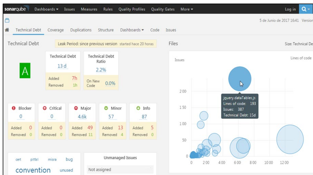
Ilustración 83 - Métricas de mantenibilidad
