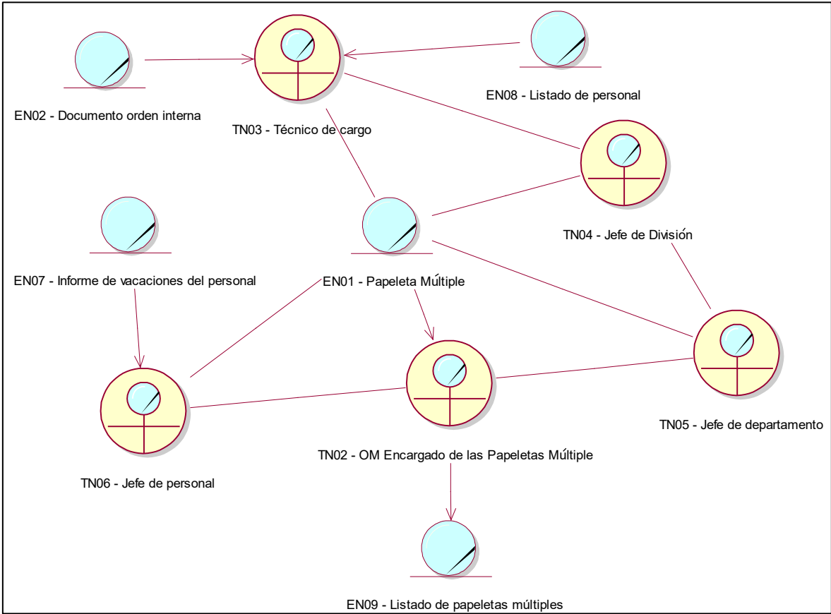
Ilustración 15 - Diagrama de clases CUN02 Fuente: Elaboración propia
