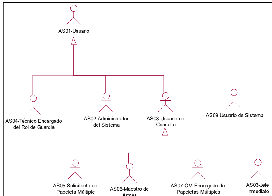
Ilustración 19 - Diagrama de Casos de Actores del Sistema Fuente: Elaboración propia
