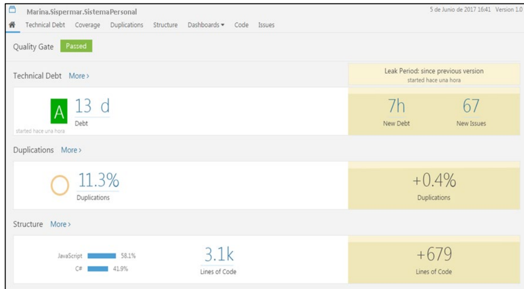
Ilustración 82 - Herramienta de SonarQube Fuente: Elaboración propia
