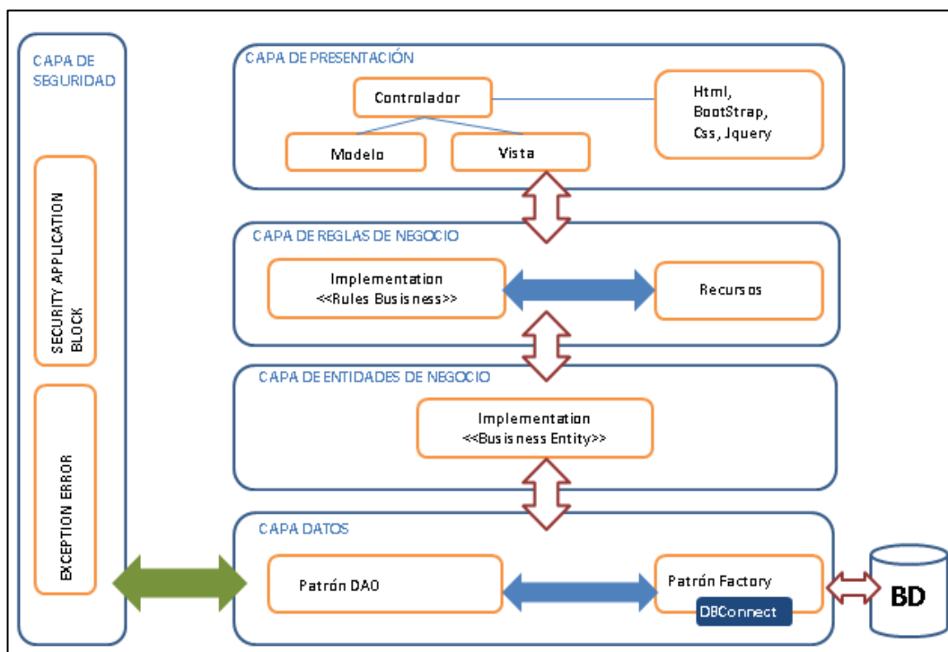
Ilustración 79- Patrón de Diseño Fuente: Elaboración propia
