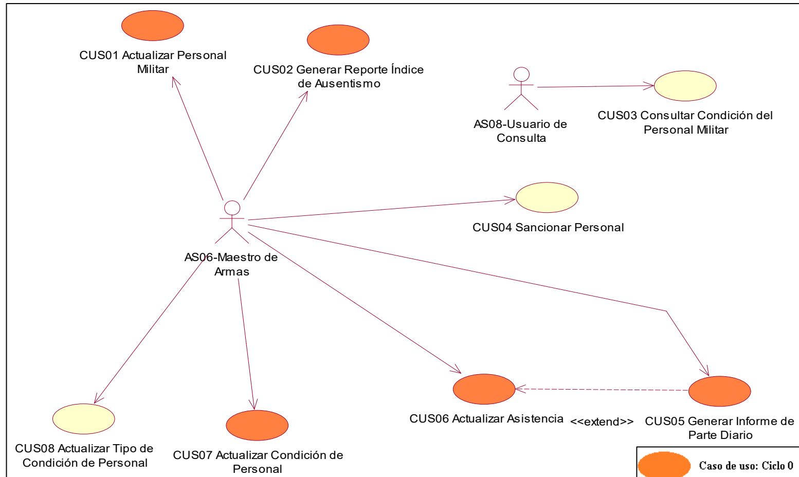
Ilustración 21 - Diagrama de caso de uso - Gestionar Condición de Personal Fuente: Elaboración propia
