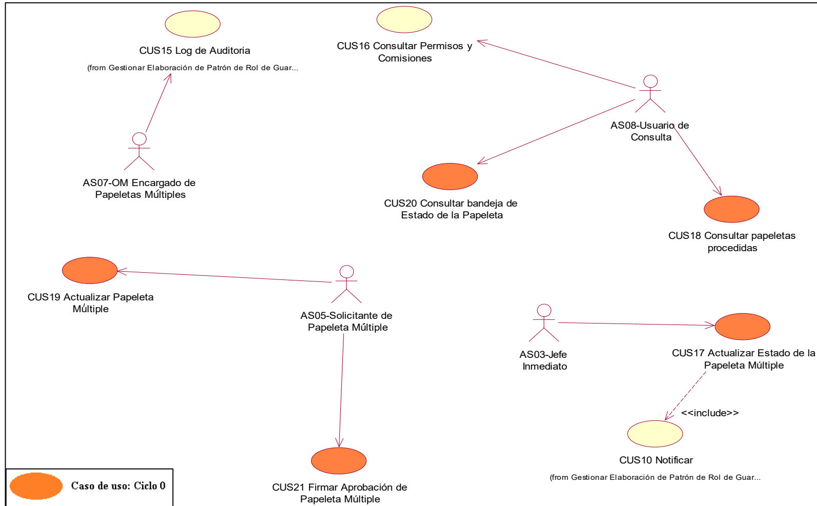
Ilustración 23-Diagrama de casos de uso de Gestionar Papeleta Múltiple
